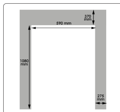
Måttskiss SU1001.
